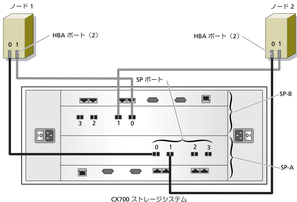
図 1-2 直接接続のファイバチャネルクラスタのケーブル接続
